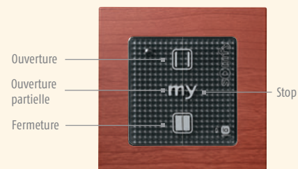
Commande pour porte battante ou latérale
